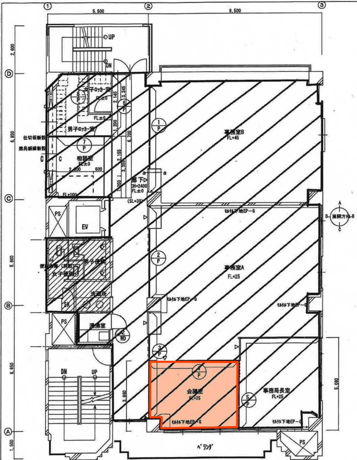
4階 平面図 1/100
